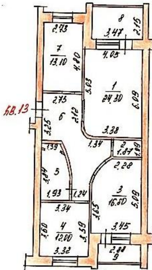
Рис.1. Поэтажный план согласно кадастрового паспорта
